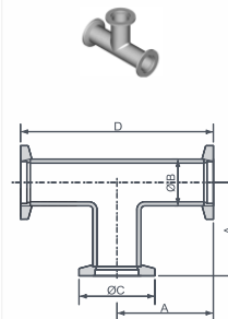
Тройник ISO-KF равнопроходный Исполнение: из нержавеющей стали
