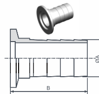
Штуцер ISO-KF с наконечником Исполнение: из нержавеющей стали под резиновые вакуумные шланги
