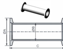
Патрубок ISO-KF Исполнение: из нержавеющей стали
