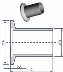
Фланец ISO-KF с длинным патрубком Исполнение: из нержавеющей стали
