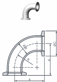
Уголок ISO-KF тянутый Исполнение: из нержавеющей стали
